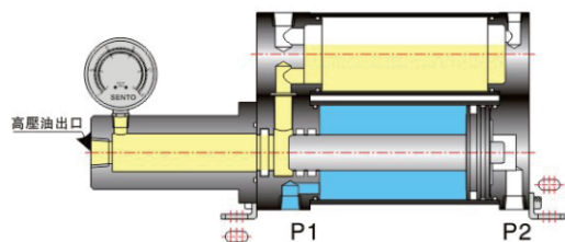
图一：P1进气，增压器处于回位状态；
