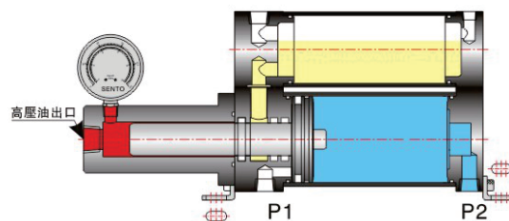
图二：P2进气，增压器产生高压油；
